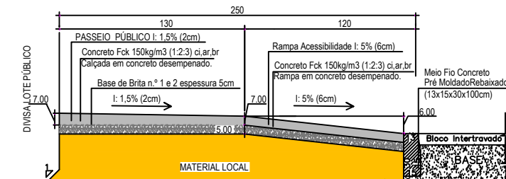
Corte Esquemático Calçadas
