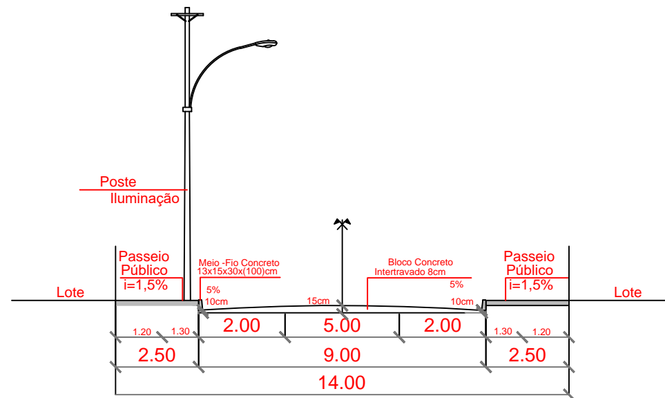
RUA CEREJEIRAS Gabarito 14,00 m Esc.: s/esc.
