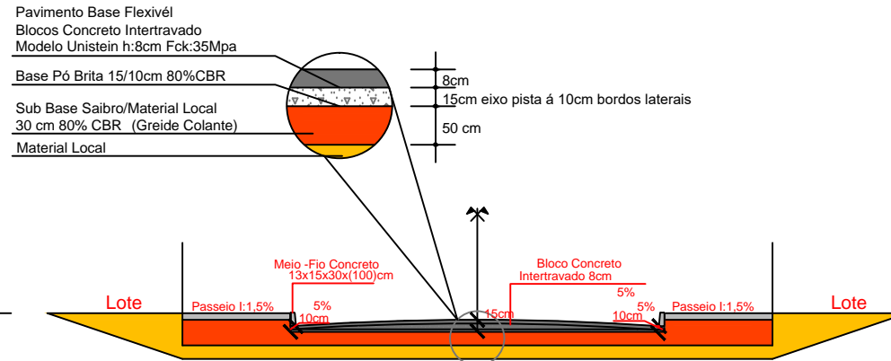
Corte Esquemático Transversal Pavimentação Greide Colante Estacas E0/E6+17m
