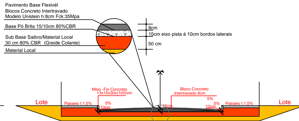
Corte Esquemático Transversal Pavimentação Greide Colante Estacas E0/E6+17m Esc.: s/esc.
