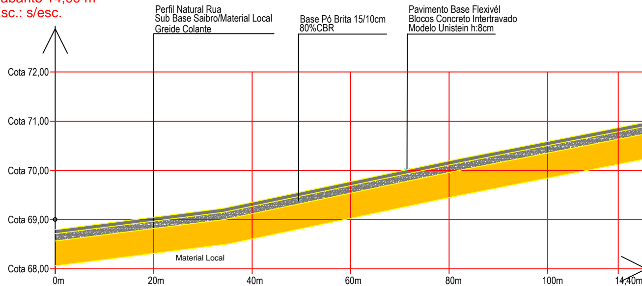
Corte Esquemático Transversal Pavimentação Greide Colante Estacas E0/E6+17m
