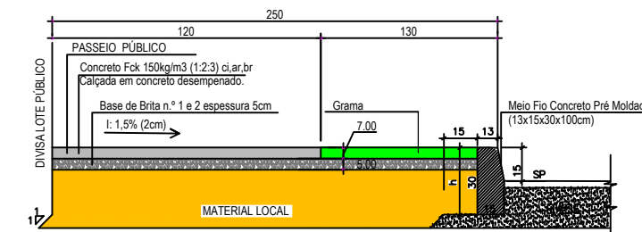
Corte Esquemático Calçadas Esc.: s/esc.
