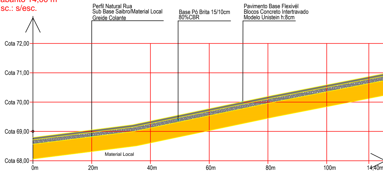
Corte Esquemático Transversal Pavimentação Greide Colante Estacas E0/E6+17m Esc.: s/esc.
