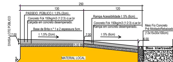
Corte Esquemático Calçadas Esc.: s/esc.
