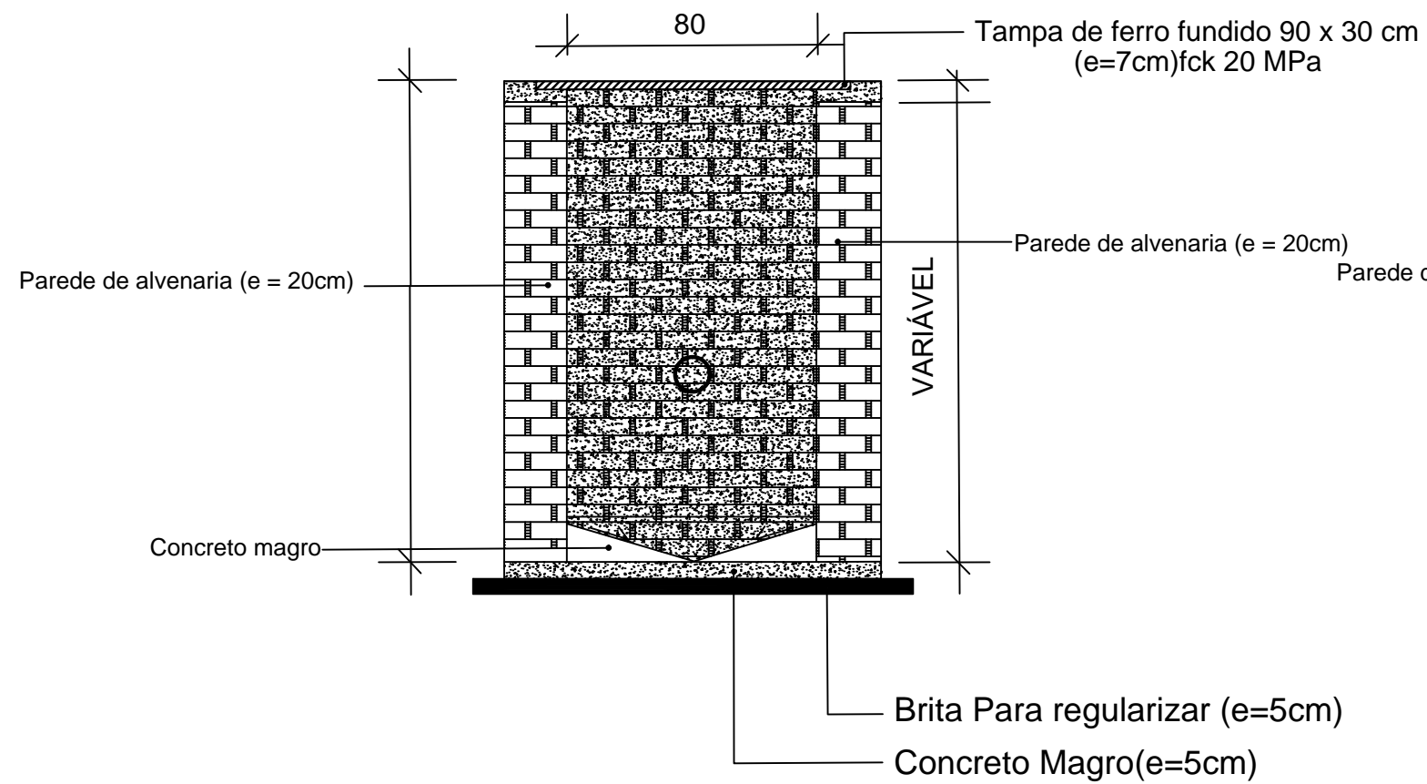
CORTE A-A'- CAIXA P/ REGISTROS (0,80x0,30) interno
