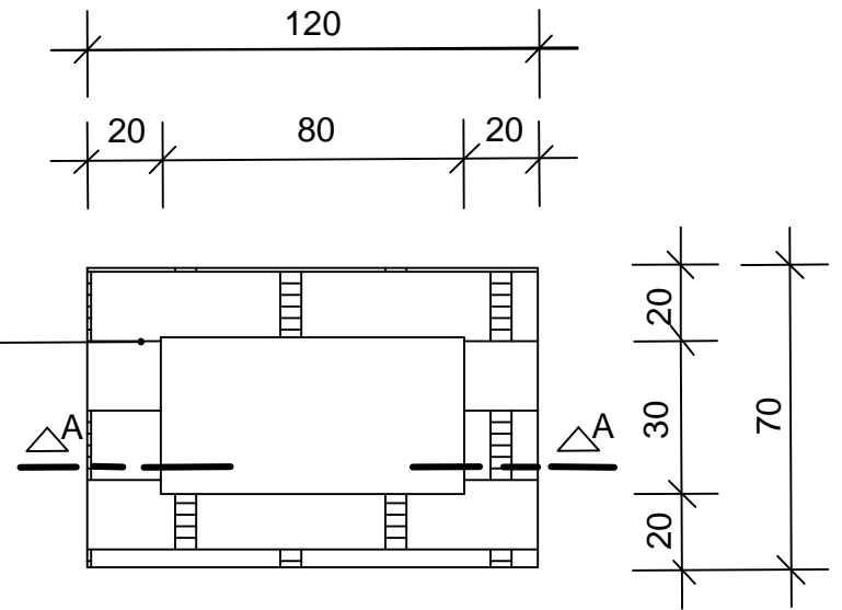
PLANTA BAIXA - CAIXA P/ REGISTROS (0,80x0,30) interno
